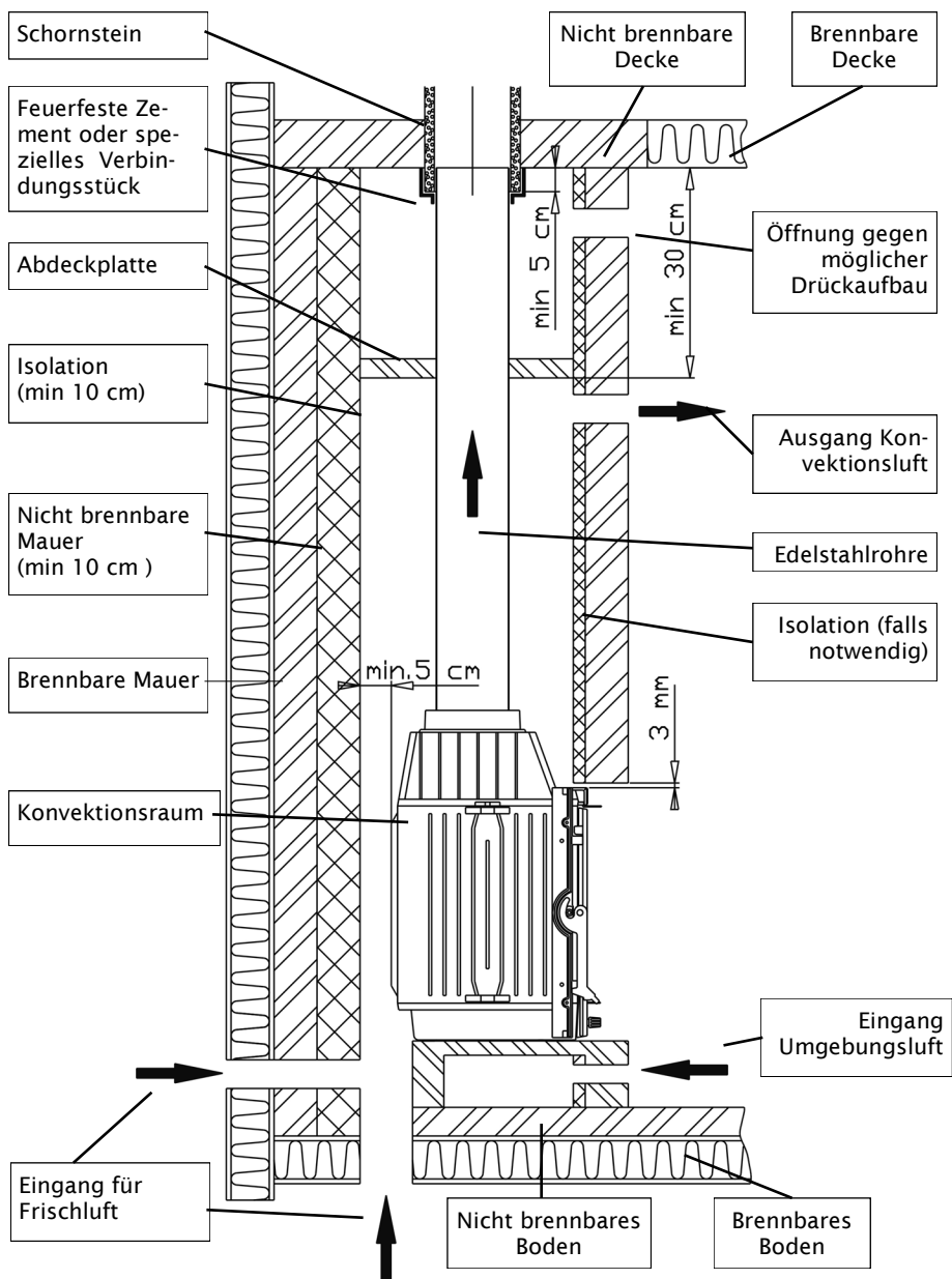
Beispiel einer Aufstellung in brennbaren Materialien
